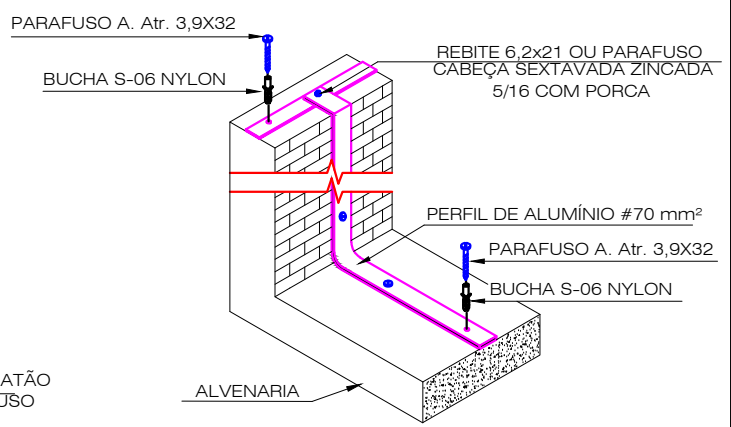
DET. 12: INTERLIGAÇÃO EM DESNÍVEL DE ALTURA ATRAVÉS DE PERFIL DE ALUMÍNIO #70mm²
