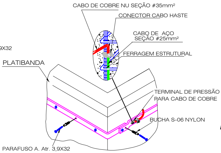
DETALHE 06: INTERLIGAÇÃO ENTRE PERFIL DE ALUMÍNIO E CABO DE COBRE DE 35 mm² NA LATERAL DA EDIFICAÇÃO
