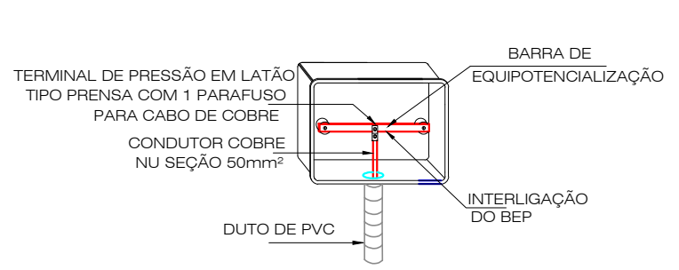
DETALHE 03: BARRA DE EQUIPOTENCIALIZAÇÃO
