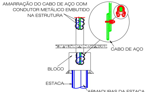
DETALHE 02: INTERLIGAÇÃO ENTRE CABO DE AÇO E FUNDAÇÃO
