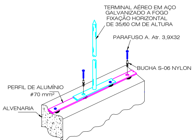
DETALHE 08: CONEXÃO COM PERFIL DE ALUMÍNIO COM TERMINAL AÉREO SOBRE A ALVENARIA
