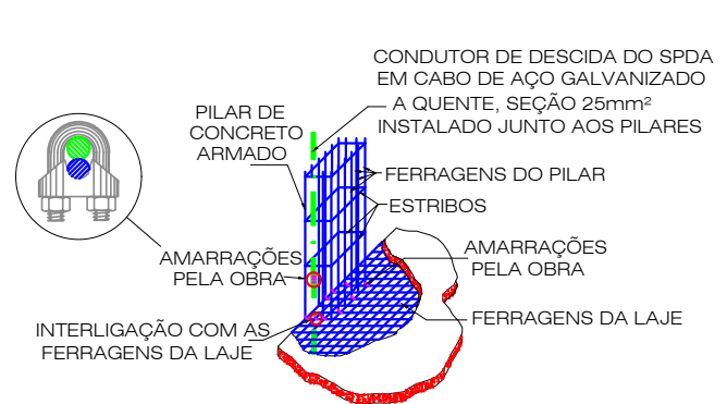
DETALHE 01: CONDUCTOR DE AÇO JUNTO ÀS ARMADURAS DA ESTRUTURA
