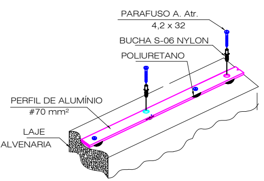
DETALHE 04: PERFIL DE ALUMÍNIO FIXADO SOBRE ALVENARIA
