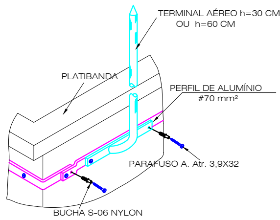
DETALHE 07: CONEXÃO DO TERMINAL AÉREO COM PERFIL DE ALUMÍNIO FIXADO NA LATERAL DA EDIFICAÇÃO
