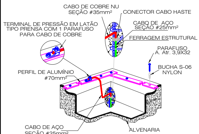
DETALHE 09: CONEXÃO COM MALHA CAPTORA CONVENCIONAL EM CABO DE COBRE NU SEÇÃO #35 mm² ÀS FERRAGENS ESTRUTURAIS DA EDIFICAÇÃO.
