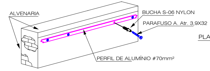
DETALHE 05: PERFIL DE ALUMÍNIO INSTALADO LATERALMENTE NA ALVENARIA.
