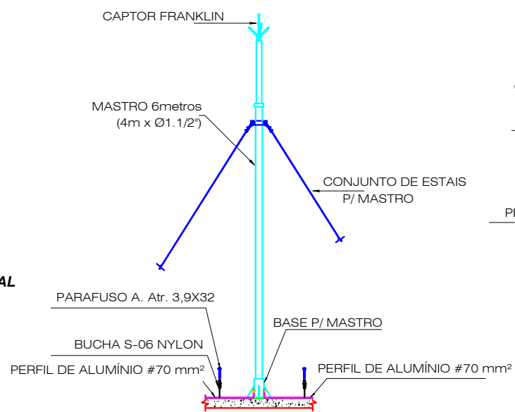
DETALHE 10: CAPTOR TIPO FRANKLIN EM MASTRO INTERLIGAÇÃO COM A MALHA CAPTORA
