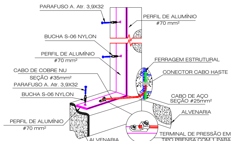
DETALHE 11: CONEXÃO DA DESCIDA COM AS (FERRAGENS ESTRUTURAIS DA EDIFICAÇÃO) E MALHA CAPTORA EM CABO DE COBRE NU SEÇÃO #35 mm²
