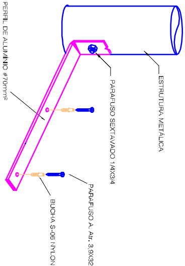
DETALHE 8: CONEXÃO COM A ESTRUTURA METÁLICA EM PERFIL DE ALUMÍNIO
