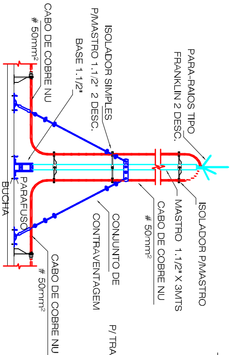
DET. 1: FIXAÇÃO PARA-RAIO TIPO FRANKLIN NA LAJE DE COBERTURA
